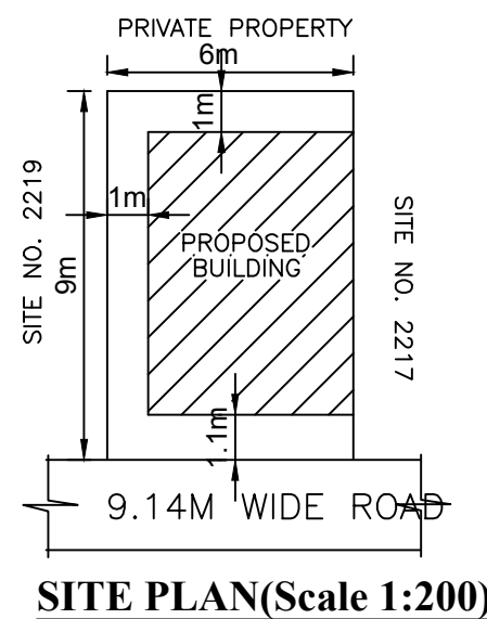
SITE PLAN(Scale 1:200)
